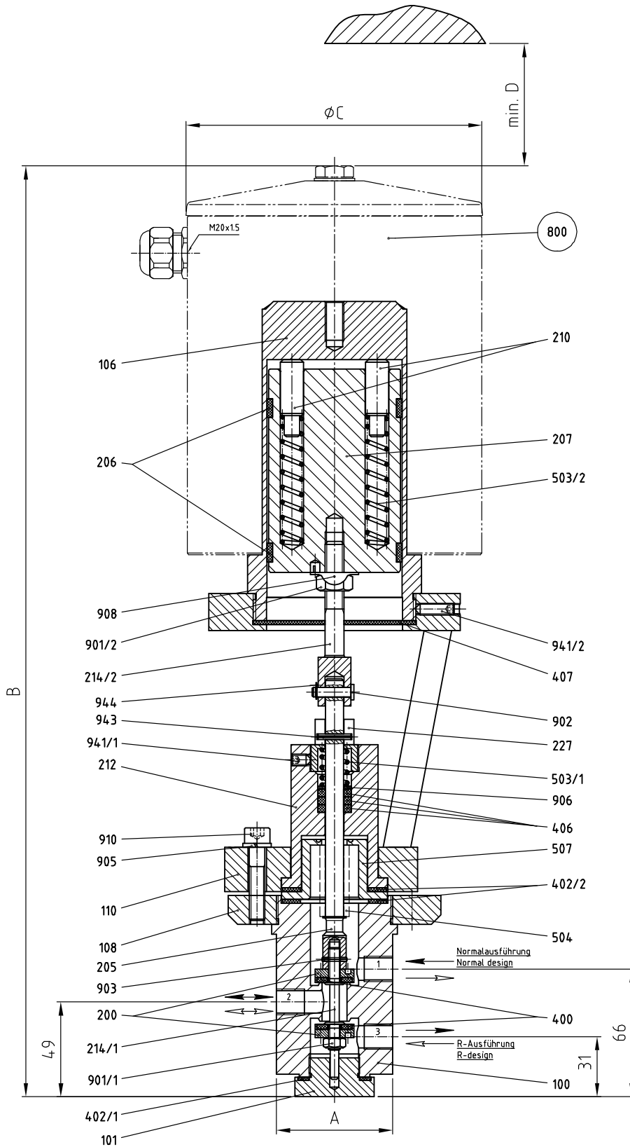
11.1 Abb. 1 Schnittzeichnung 12-EVDF 2/3/5R.(Xn).. ( G1/4, 3/8, 1/2)
