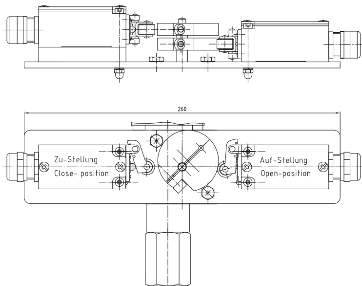
Abb.9 MRK Ma... Ausführung mit eingezogenem Durchgang
