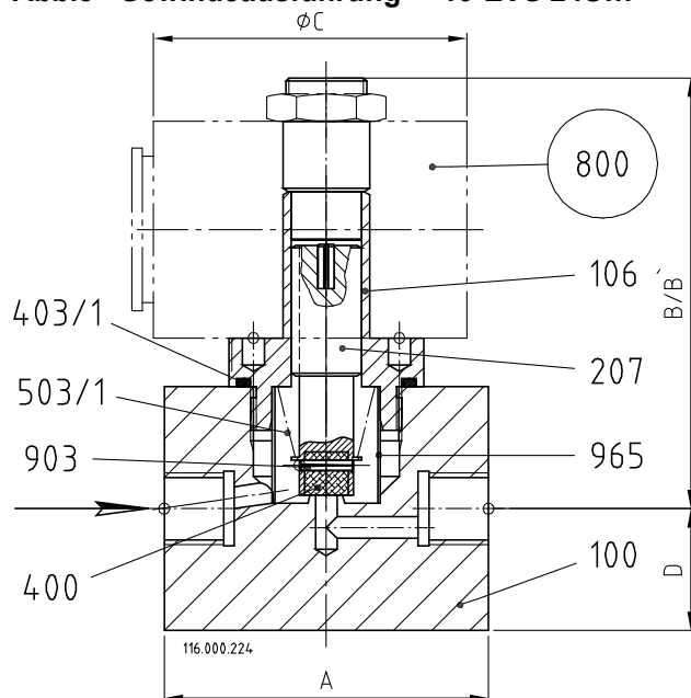
Abb.3 Gewindeausführung 10-EVS 24Ü...
