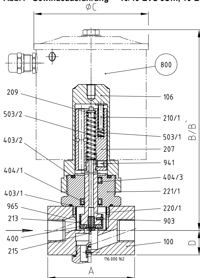
Abb.4 Gewindeausführung 10/40-EVS 5Ü..., 10-EVS 3Ü...
