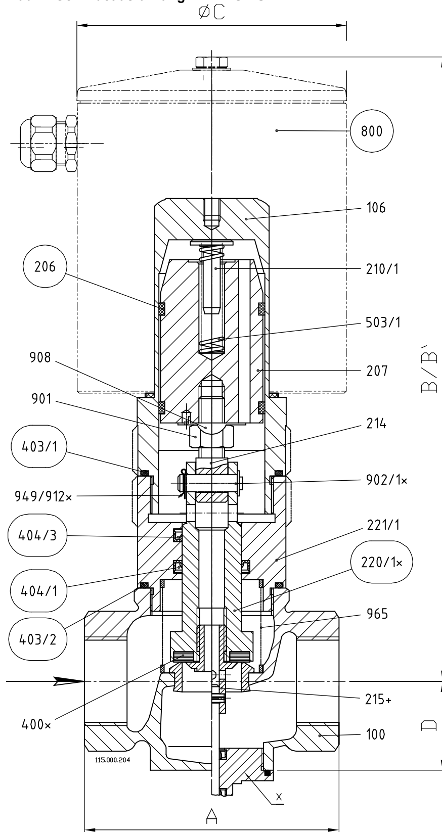
Abb.2 Gewindeausführung 4-EVS...Ü...
