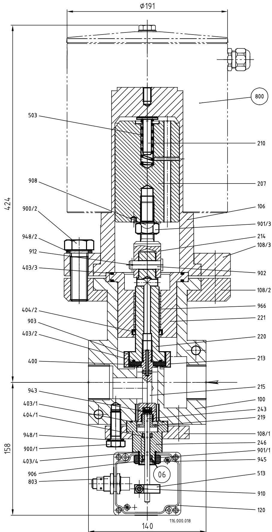
Abb. 4 120-EVS 5...; 135-EVS 12/10..
