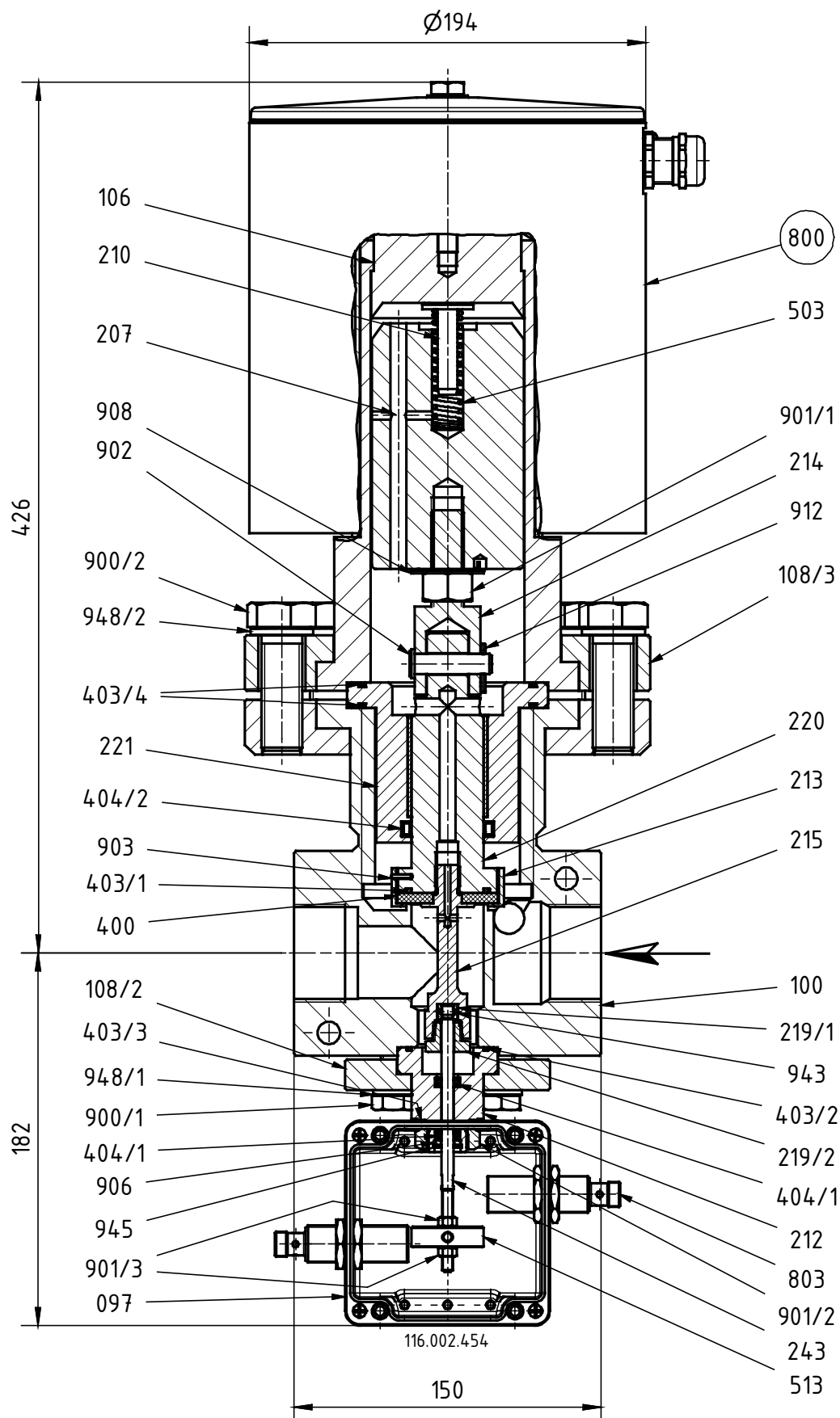
Abb. 5 135-EVS 15.., 160-EVS 15..
