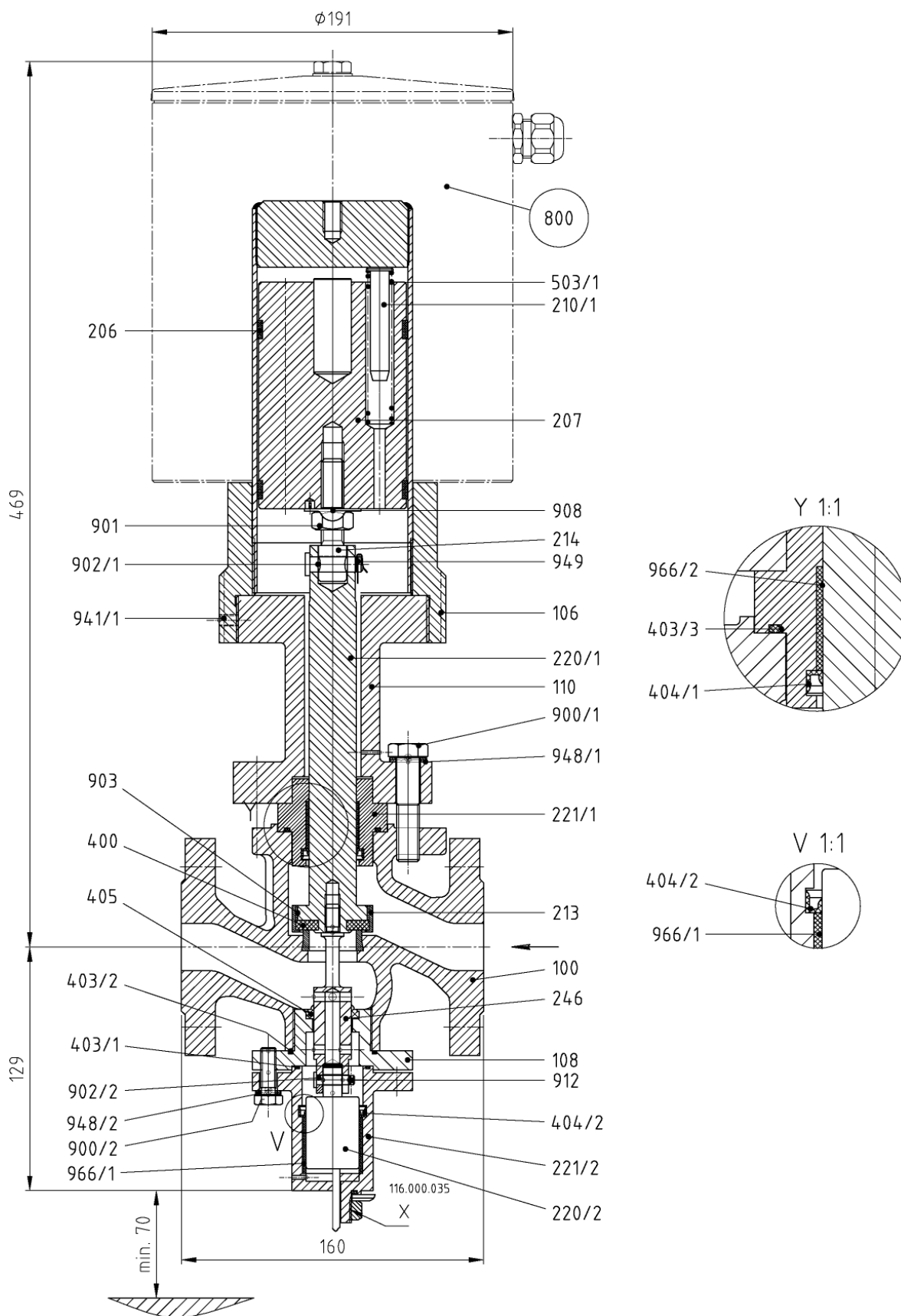
Abb. 2 40-EVS..N(H)
