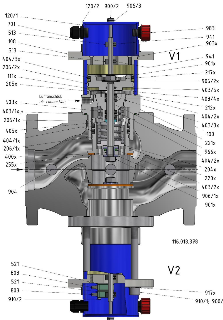
Abb.3 Schnittzeichnung PXI...
