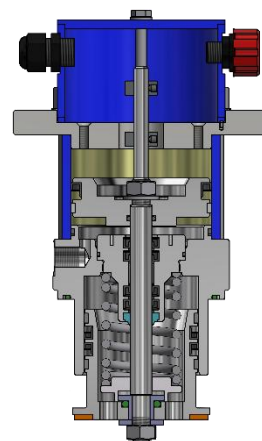
Abb.2b Dichteinheit
