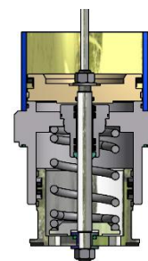
Abb.3 Schnittzeichnung PXI...
