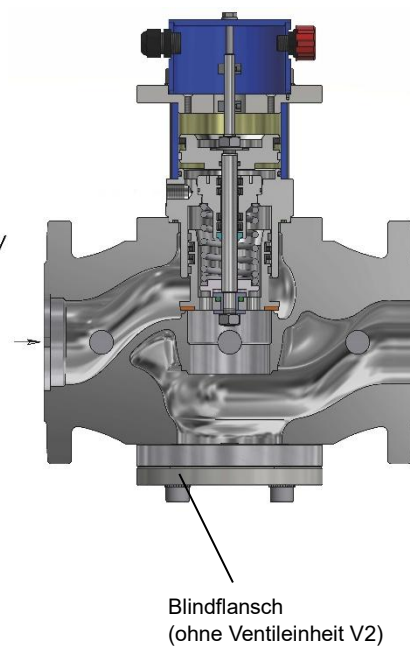
Abb.3 Schnittzeichnung PXI...
