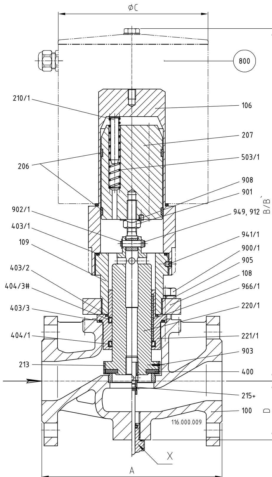
Abb.3 Flanschausführung 40-EVSA 5NH...
