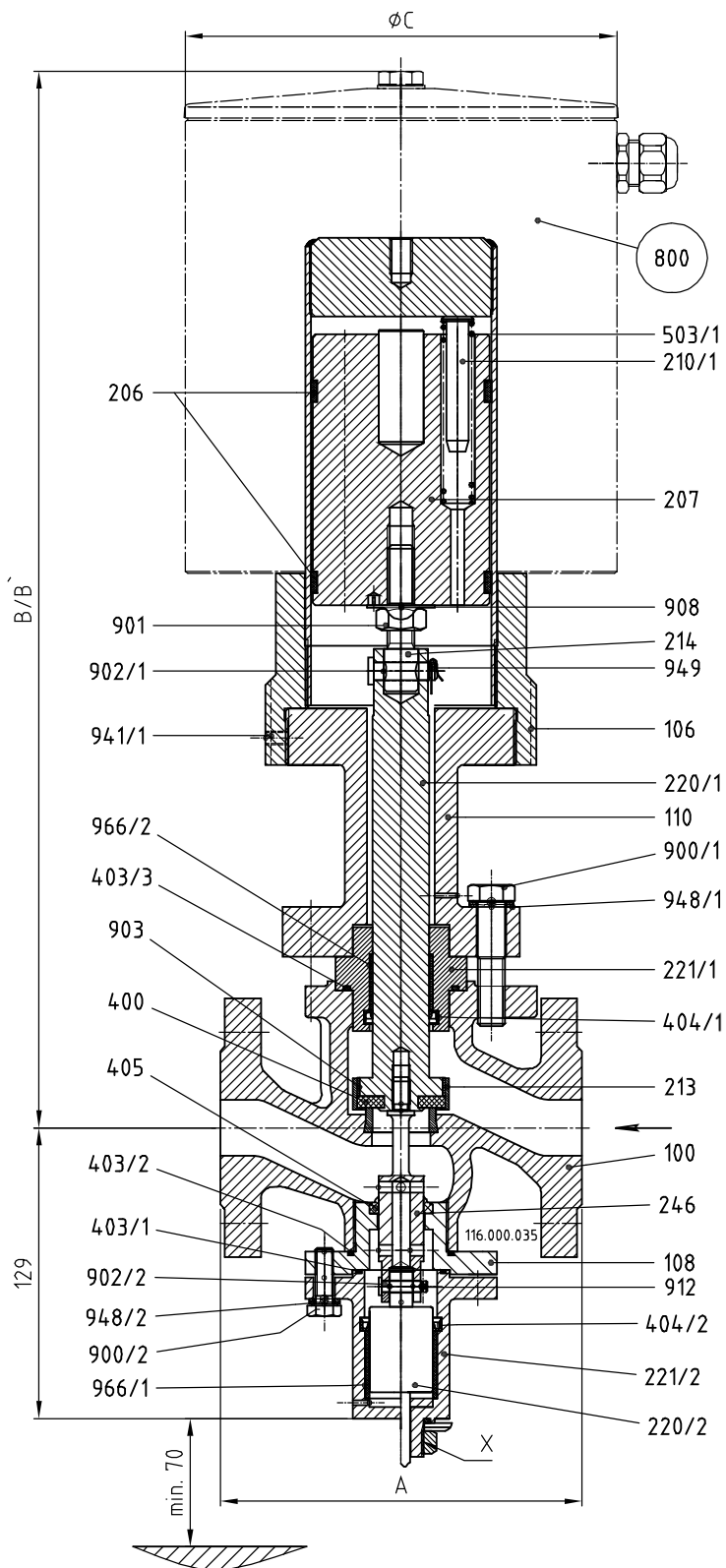
Abb.4 Flanschausführung 40-EVSA 10NH
