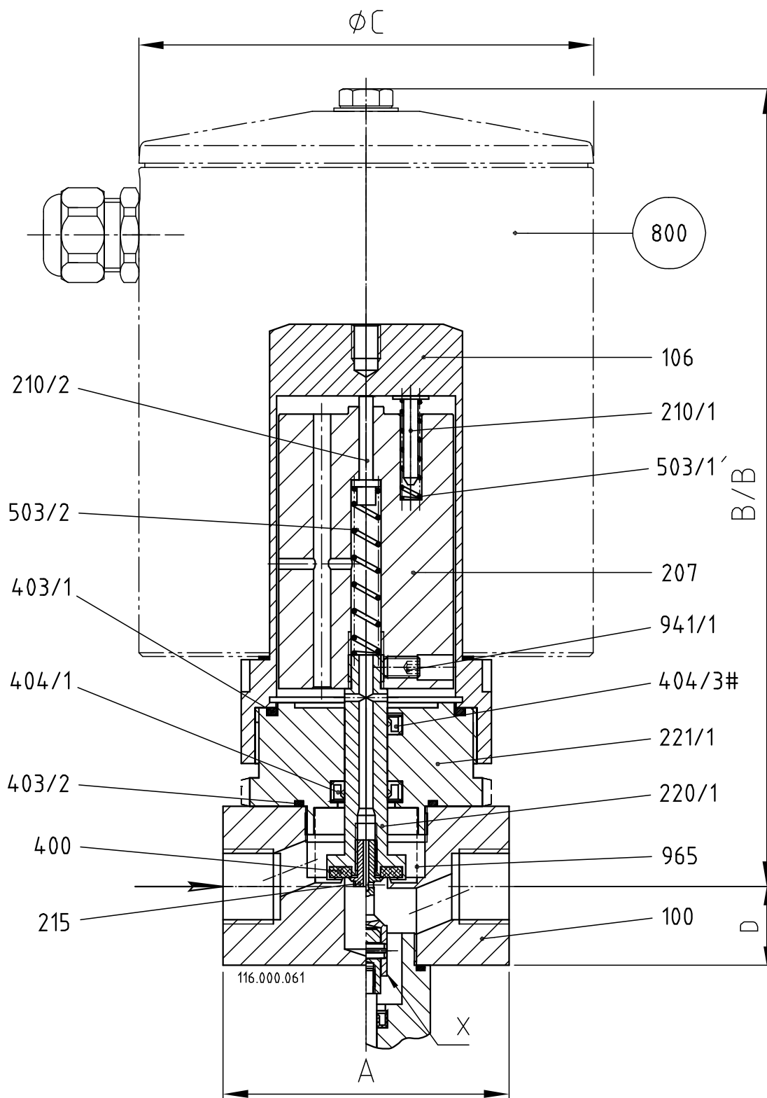
Abb.7 Gewindeausführung 40-EVSA-5-4
