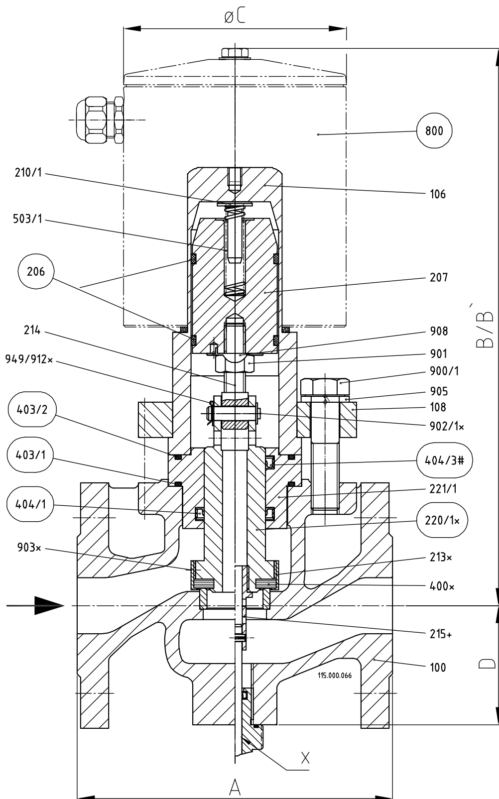
Abb. 1 Flanschausführung 4/10-EVSA 16-EVSA 30N(H)
