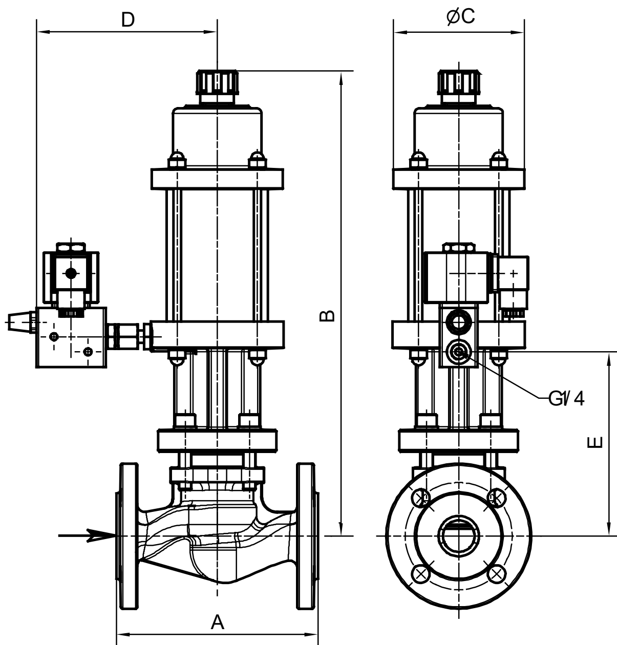
Abb. 3 Ansichtszeichnung ...-4-EPVA...N(H).. bei Abb. 2
