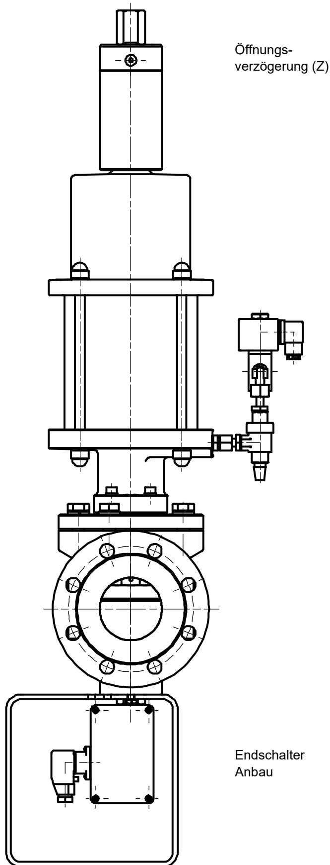
Abb. 4 Ansichtszeichnung sonder ...EPVA...(N)H.-4.Z.. + Ends.-Anb.
