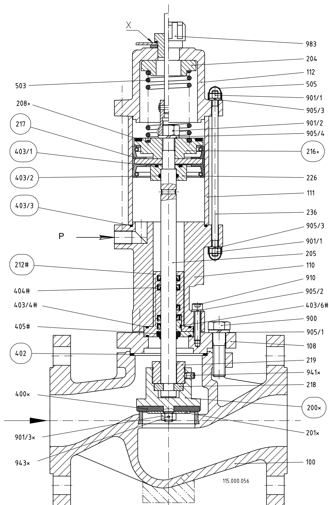
Abb. 5 Schnittzeichnung
