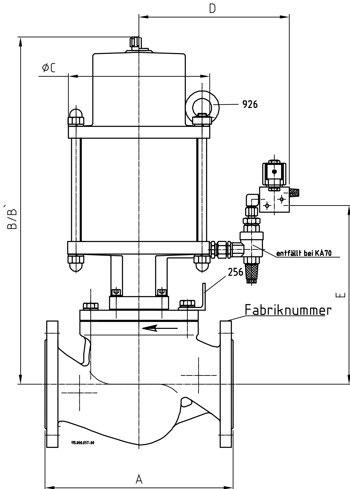
Abb. 1 Ansichtszeichnung A-Ausführung
