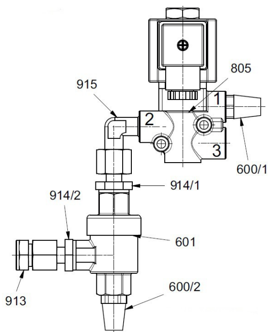
Abb. 9 Steuerventil ab KA 120
