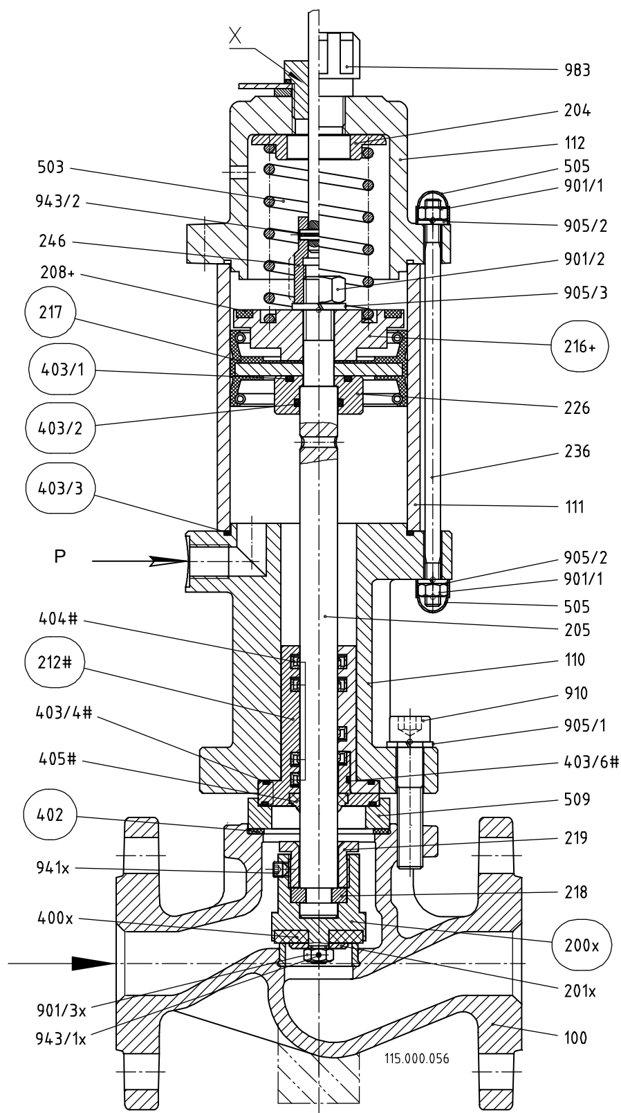
Abb. 6 Schnittzeichnung
