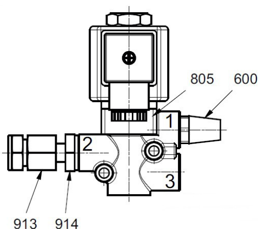
Abb. 9 Steuerventil ab KA 120
