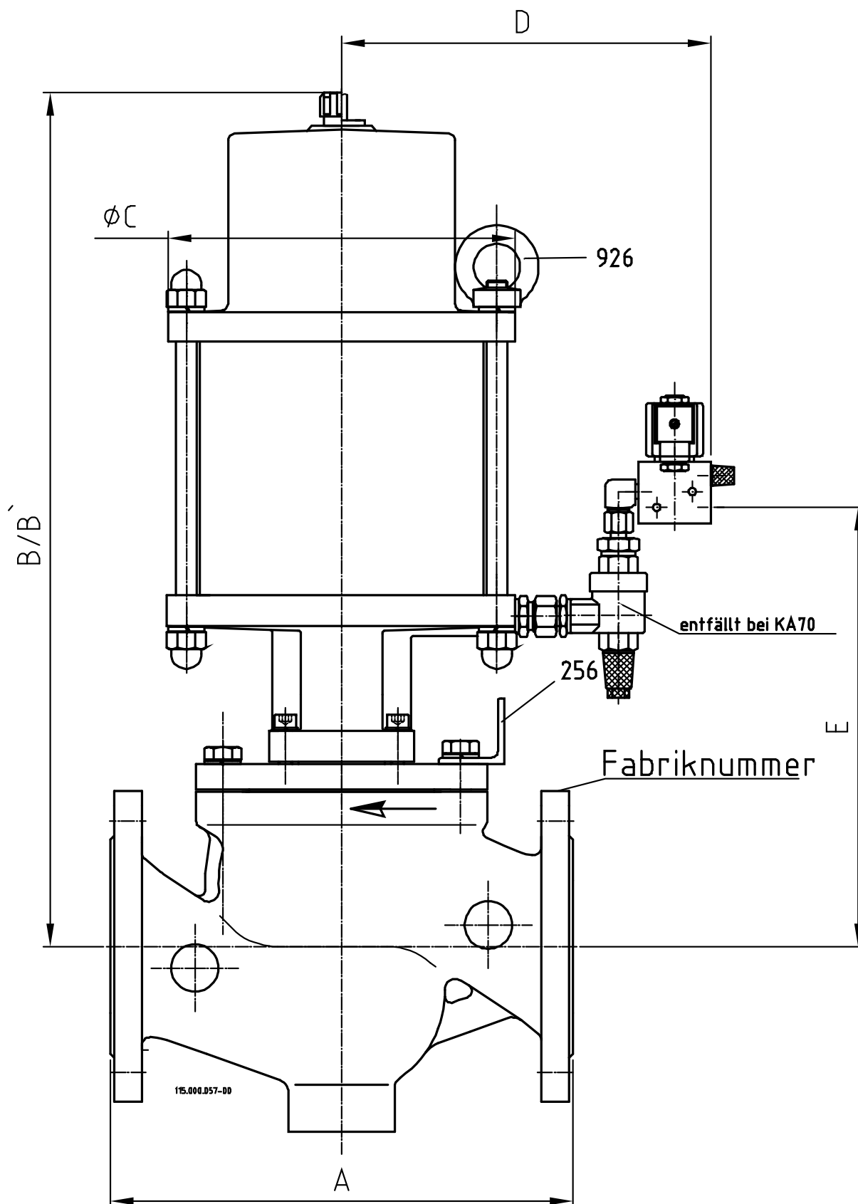
Abb. 2 Ansichtszeichnung H-Ausführung
